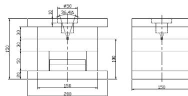
标准模架 Standard mold set
