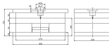
最大模架 Max mold set
