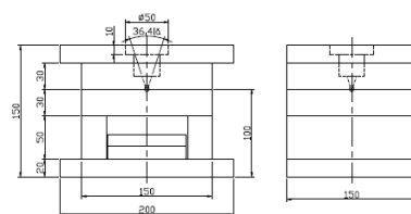
标准模架 Standard mold set
